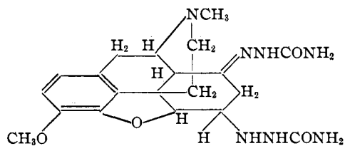
I. Pseudocodeinone semicarbazino-semicarbazone
